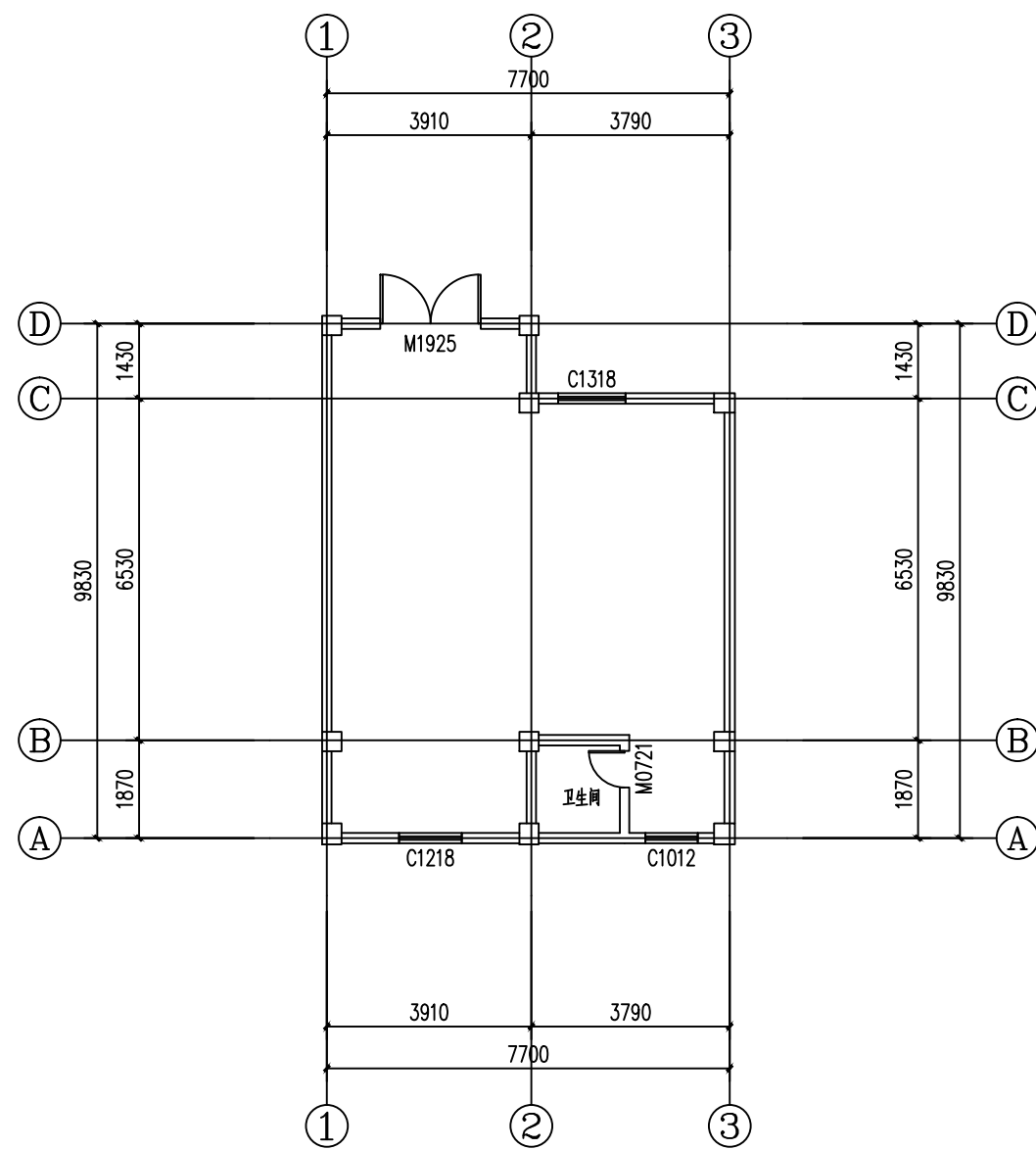
平面图 1:100 净高: 2.86m
