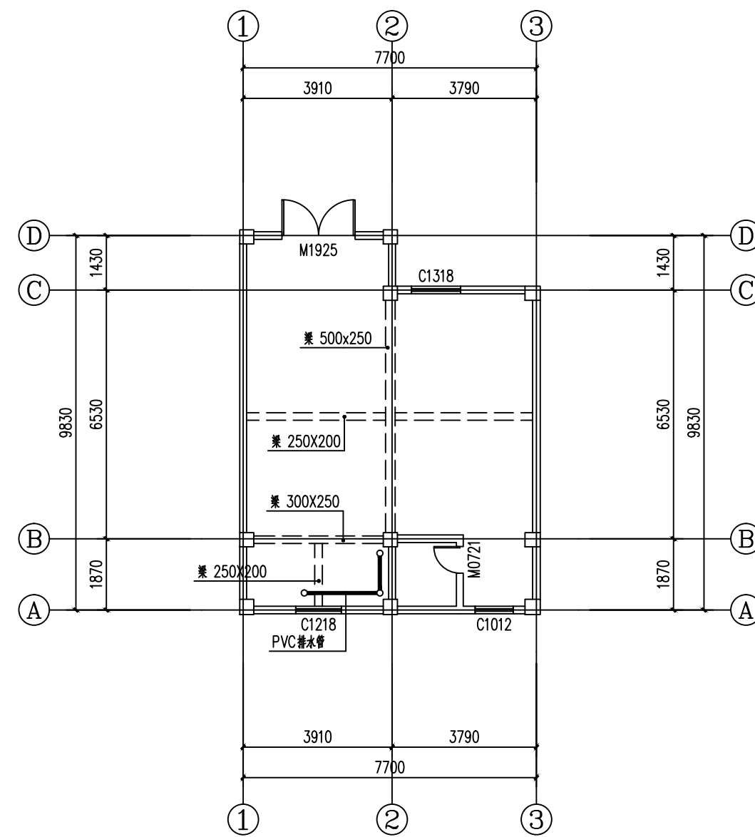
梁平面图 1:100 净高: 2.86m
